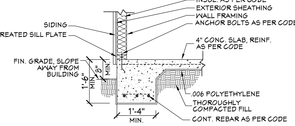
206 FTG. DET.
