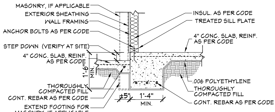
205 FTG. DET.
