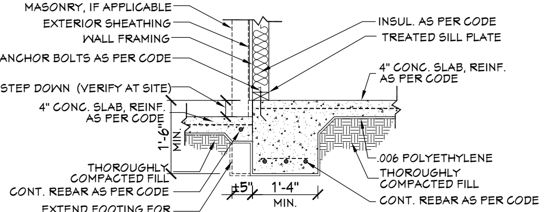
205 FTG. DET.
