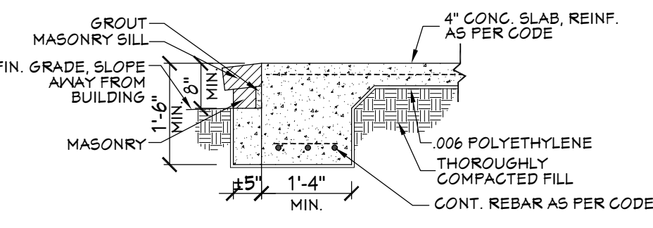
207 FTG. DET.
