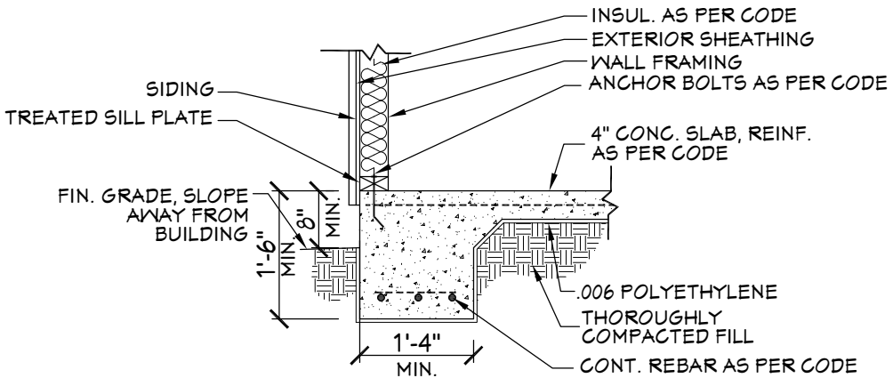
206 FTG. DET.
