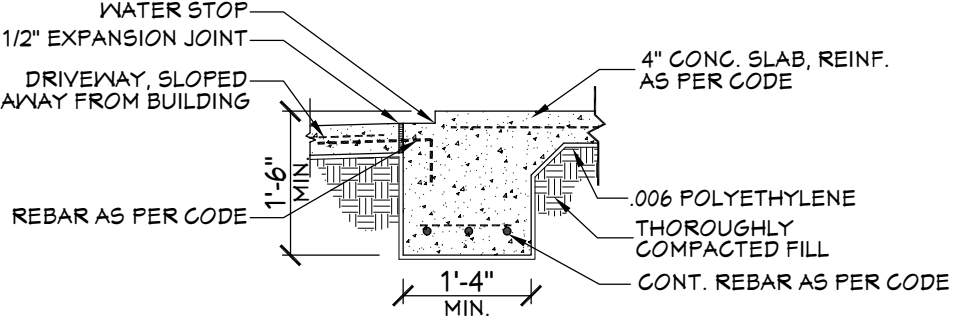
202 FTG. DET.
