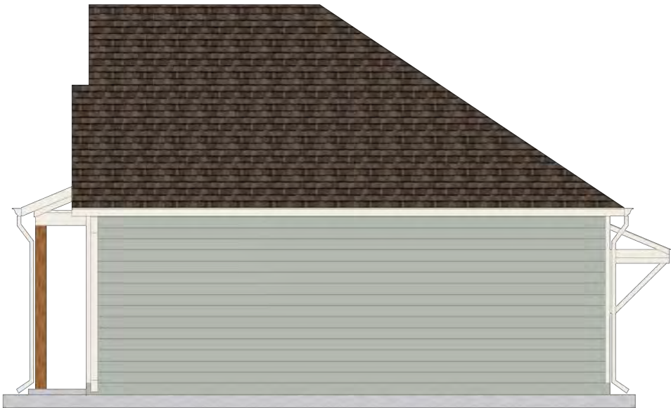
RIGHT ELEVATION
